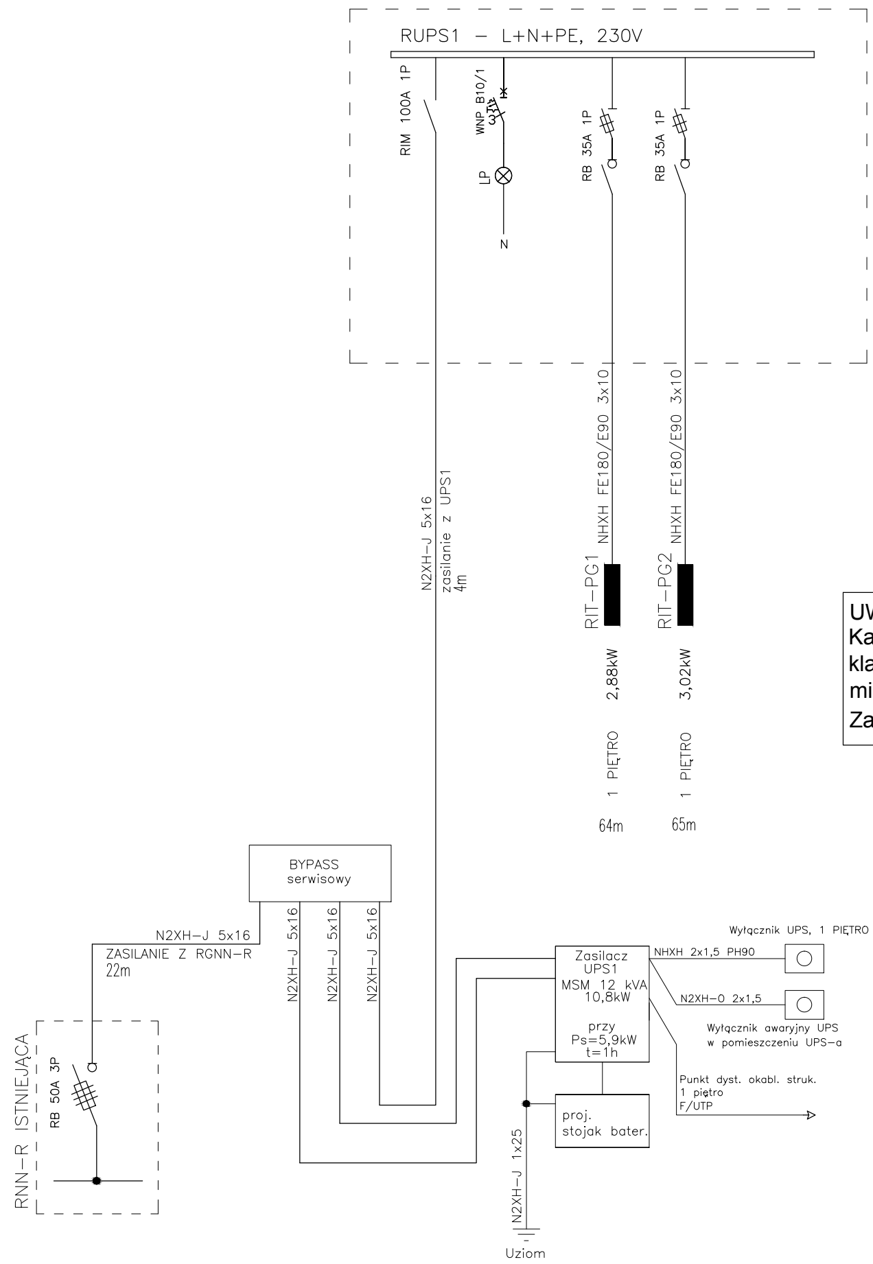
ROZDZIELNICA NATYNKOWA 300x450x150 [mm] 1x18 MOD.
